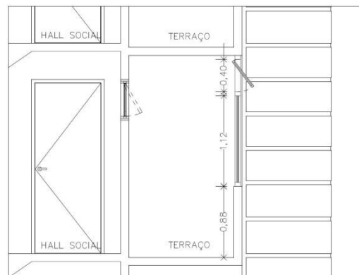
Figura 2: Corte esquemático
